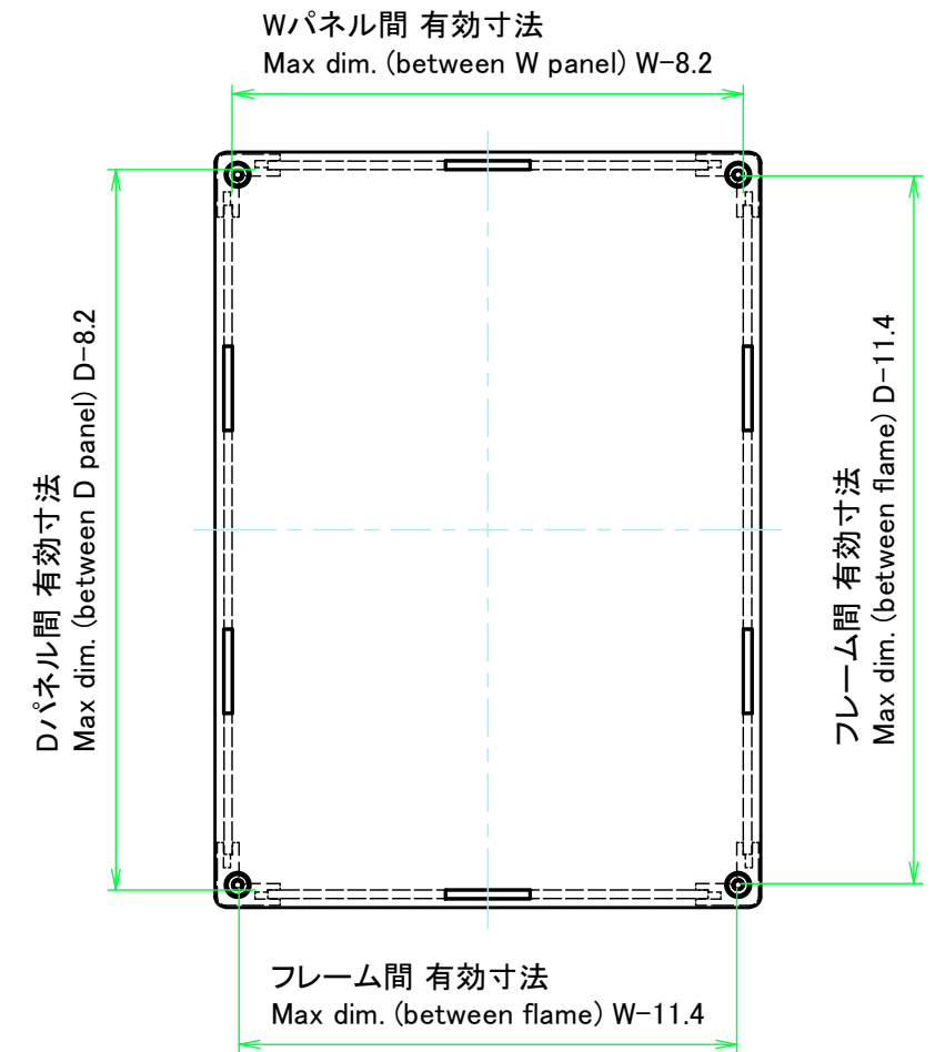
下カバー / Bottom cover
